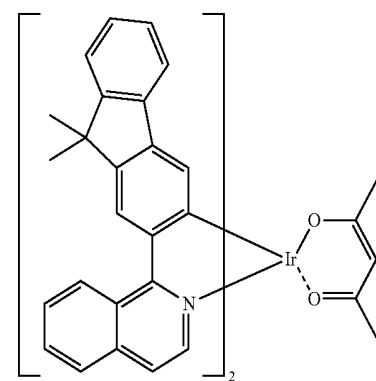
Ir(fliq) 2 (acac)
