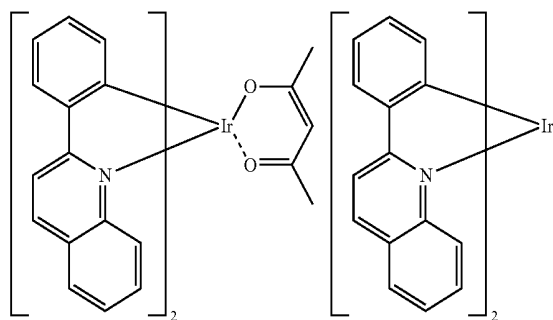
Ir(pq) 2 (acac)
