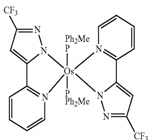
Os(fppz) 2 (PPh 2 Me) 2
