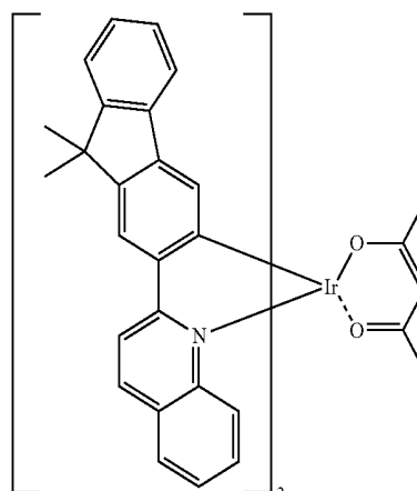
Ir(flq) 2 (acac)
