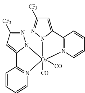
Os(fppz) 2 (CO) 2
